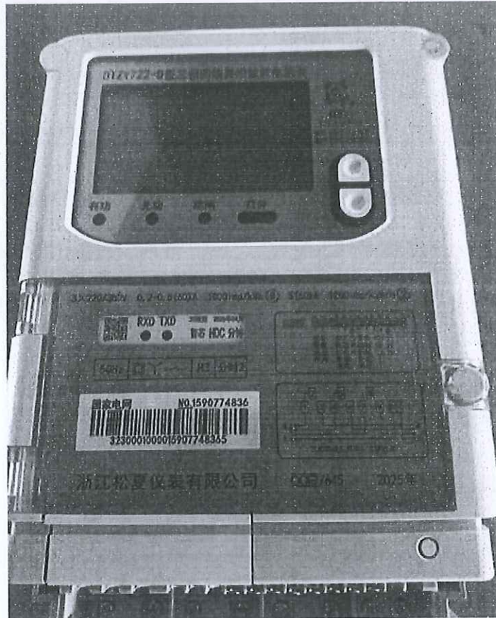
三相费控智能电能表 (DTZY722-D)
