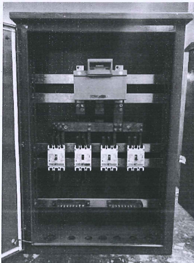
低压电缆分支箱（DFW）
