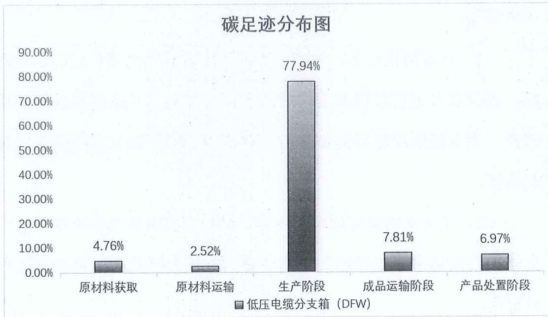
图 5.2.1.2 低压电缆分支箱 (DFW) 生命周期阶段碳排放分布图
