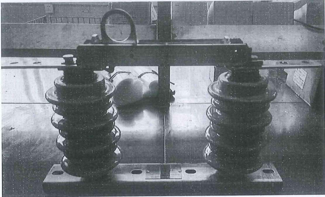
12kV 户外高压隔离开关 (HGW9-12/630-20)
