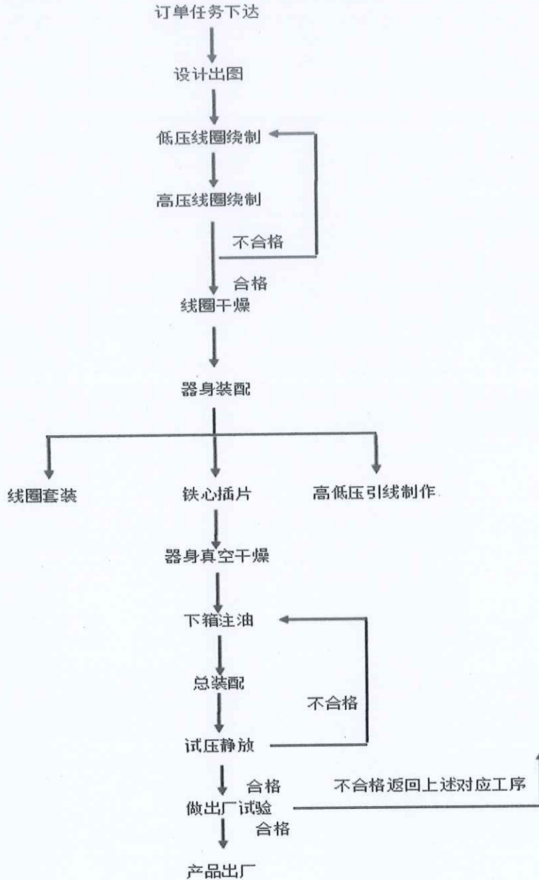
油浸式变压器生产制造工艺流程图
