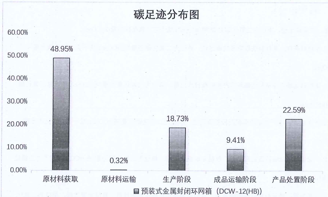
图 5.2.1.2 预装式金属封闭环网箱 (DCW-12(HB)) 生命周期阶段碳排放分布图
