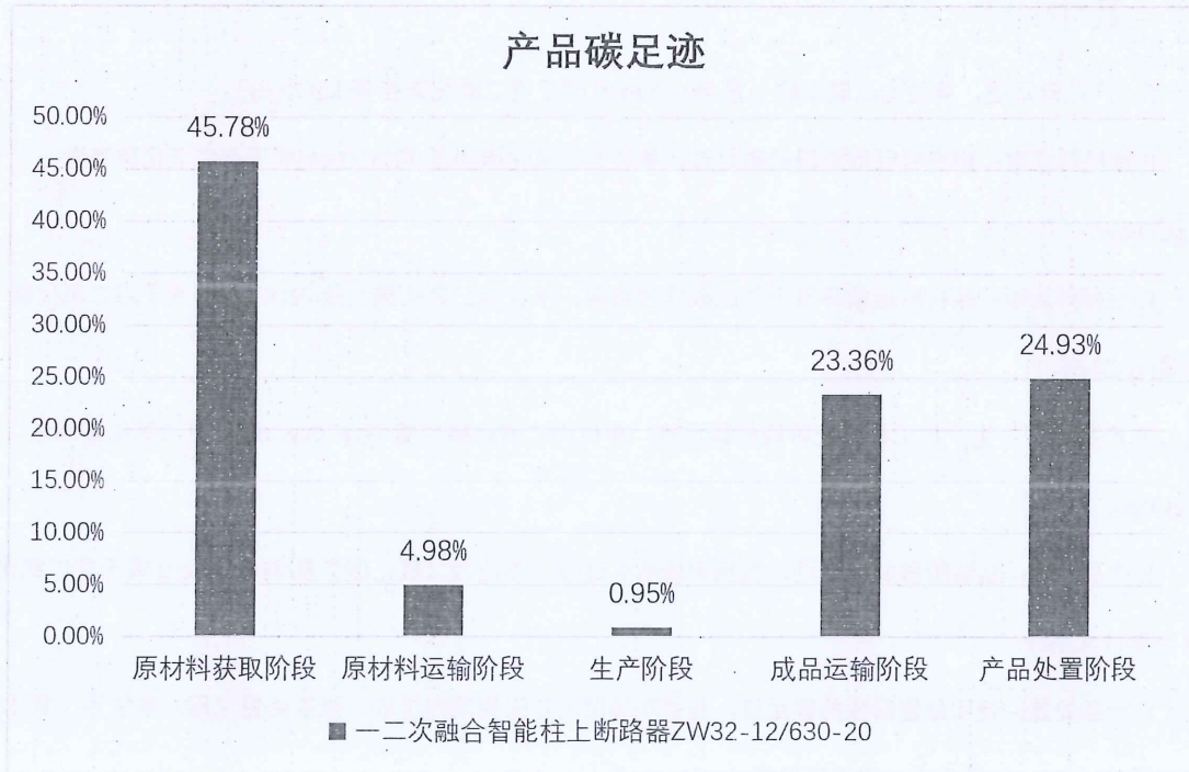
图 5.2.2 一二次融合智能柱上断路器（ZW32-12/630-20）生命周期阶段碳排放分布图
