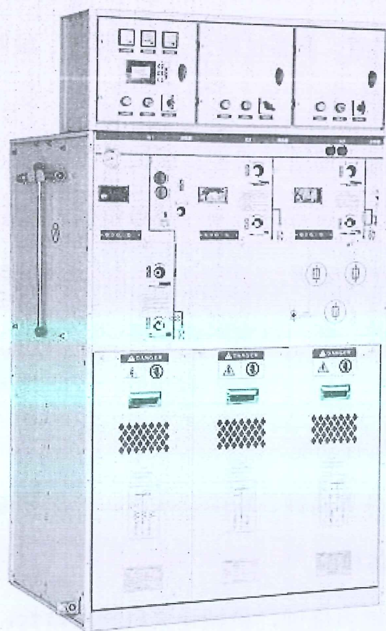
环保气体绝缘金属封闭开关设备（ZTHB-12(C)/630-20）
