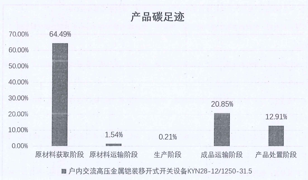
图 5.2.2 户内交流高压金属铠装移开式开关设备（KYN28-12/1250-31.5）生命周期阶段碳排放分布图
