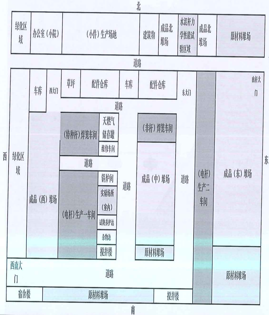
厂区平面图
