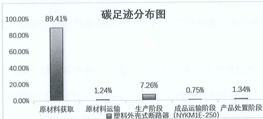
图 5.2.1.2 塑料外壳式断路器 (NYKM1E-250) 生命周期阶段碳排放分布图
