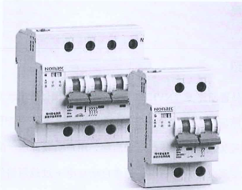
电能表外置断路器（NYKB7-W80）
