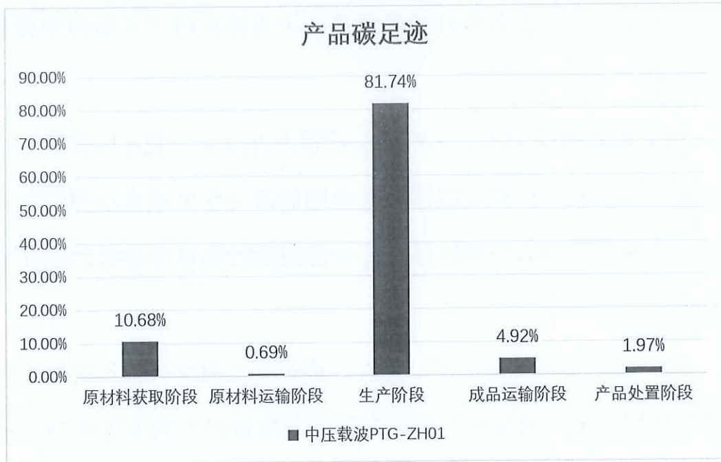
图 5.2.2 中压载波 (PTG-ZH01) 生命周期阶段碳排放分布图
