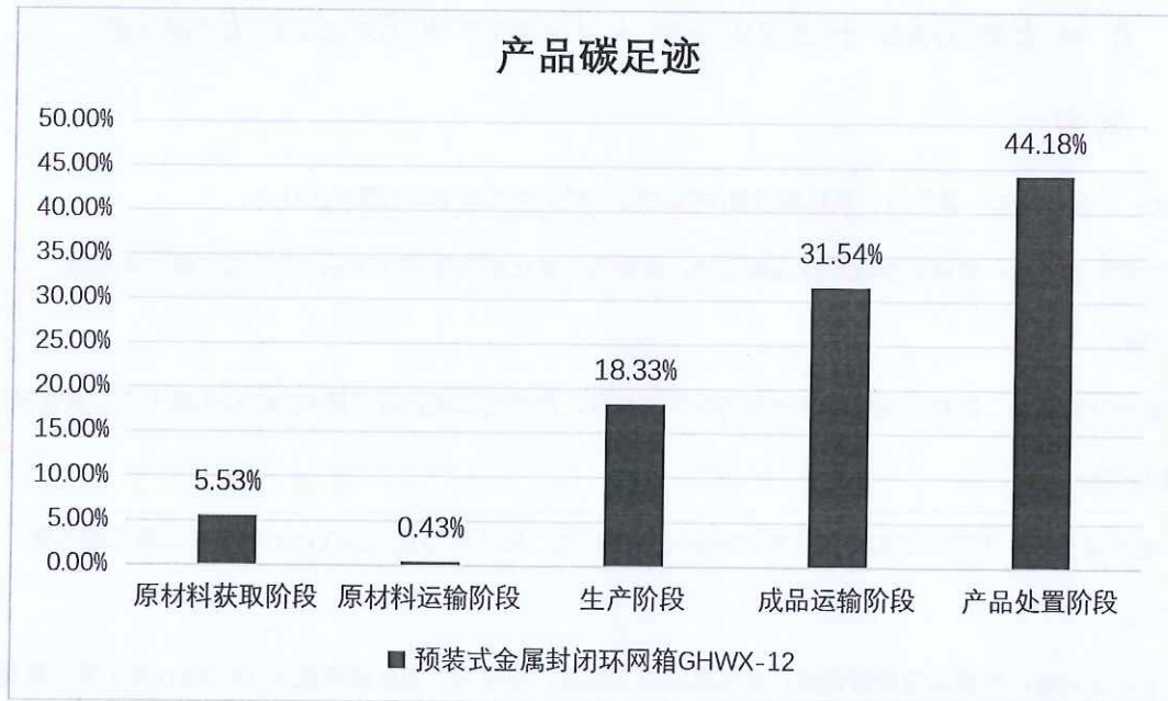
图 5.2.2 预装式金属封闭环网箱 (GHWX-12) 生命周期阶段碳排放分布图
