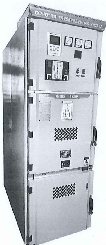
户内交流高压金属铠装移开式开关设备 (KYN28-12/1250-31.5)
