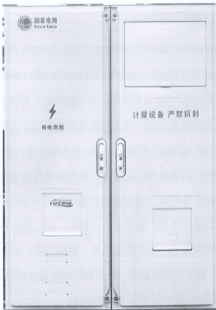
三相多表位金属计量箱 (BXS2)
