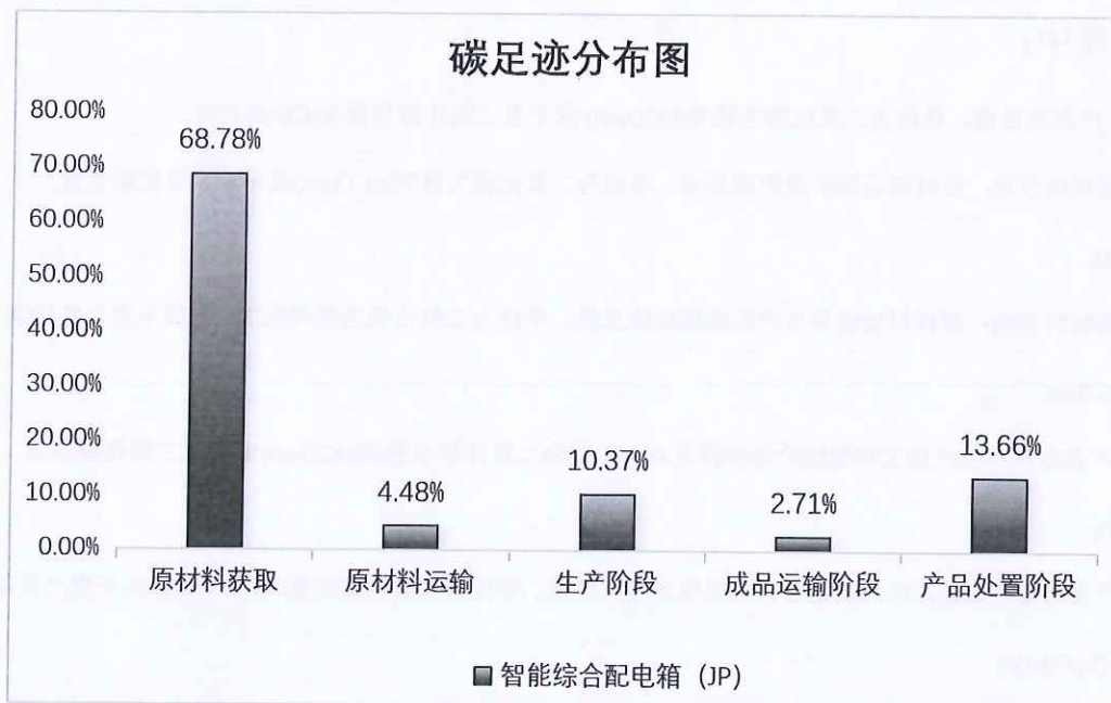
图 5.2.1.2 智能综合配电箱（低压成套开关设备）（JP）生命周期阶段碳排放分布图
