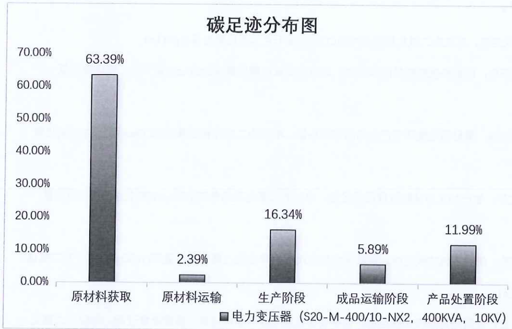
图 5.2.1.2 电力变压器 (S20-M-400/10-NX2, 400KVA, 10KV) 生命周期阶段碳排放分布图
