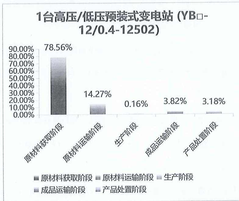
图 5.2-2 一台高压/低压预装式变电站（YB□-12/0.4-1250）
