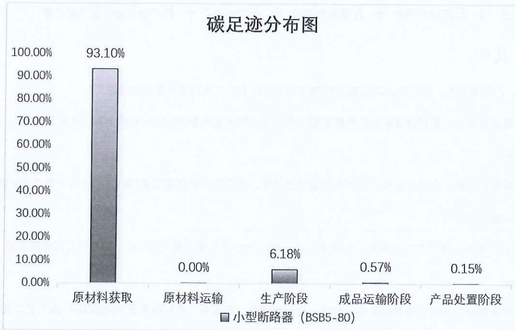
图 5.2.1.2 小型断路器 (BSB5-80) 生命周期阶段碳排放分布图
