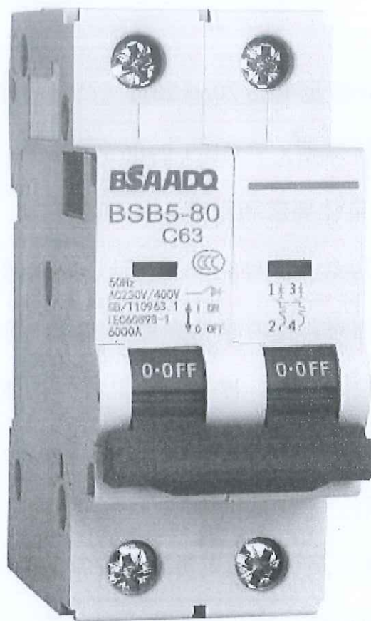
小型断路器 (BSB5-80)
