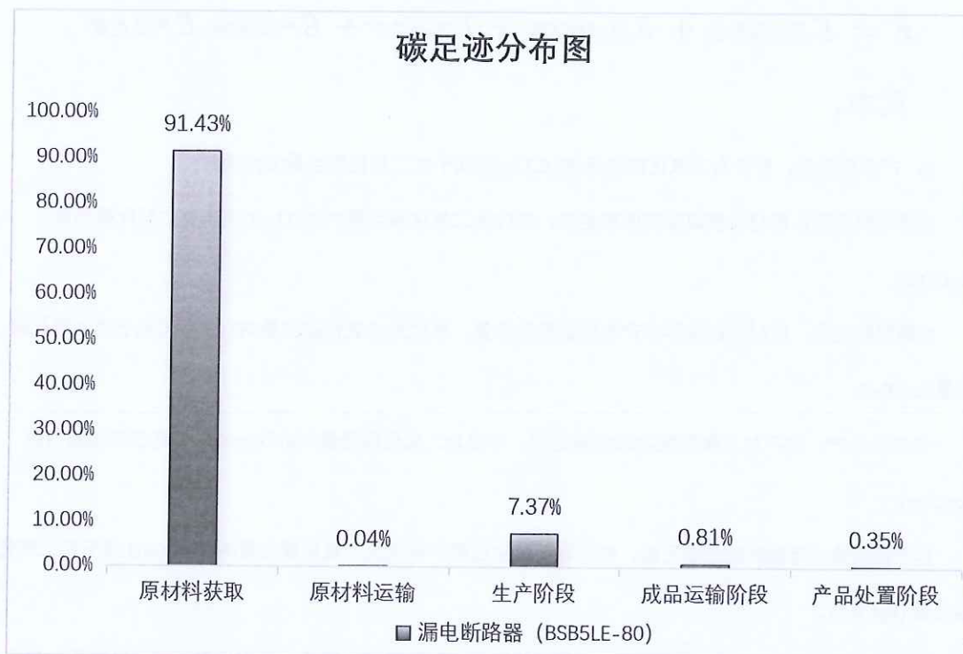
图 5.2.1.2 漏电断路器 (BSB5LE-80) 生命周期阶段碳排放分布图
