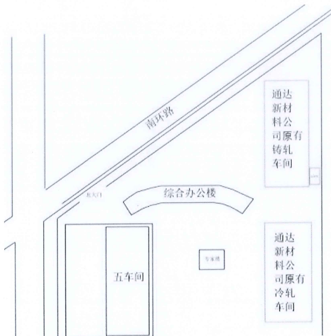
厂区布局图
