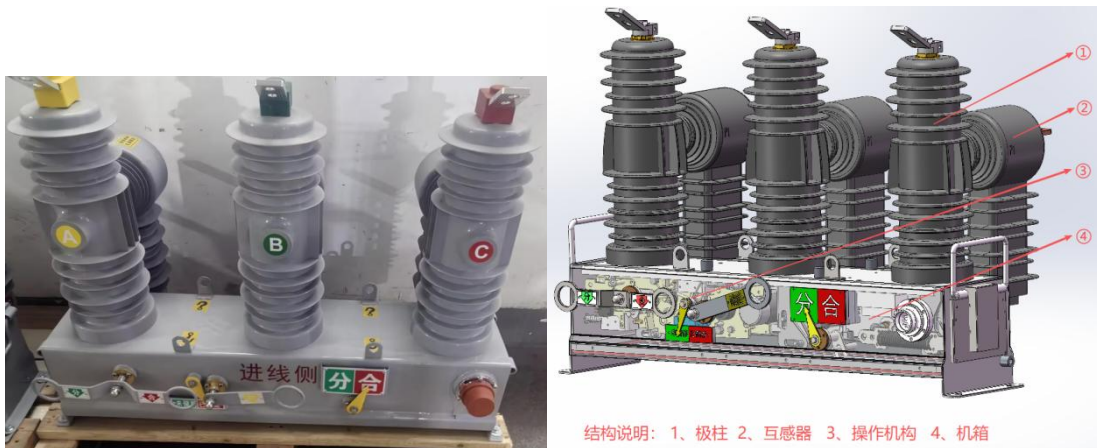
户外高压真空断路器：ZW32-12/T630-20
