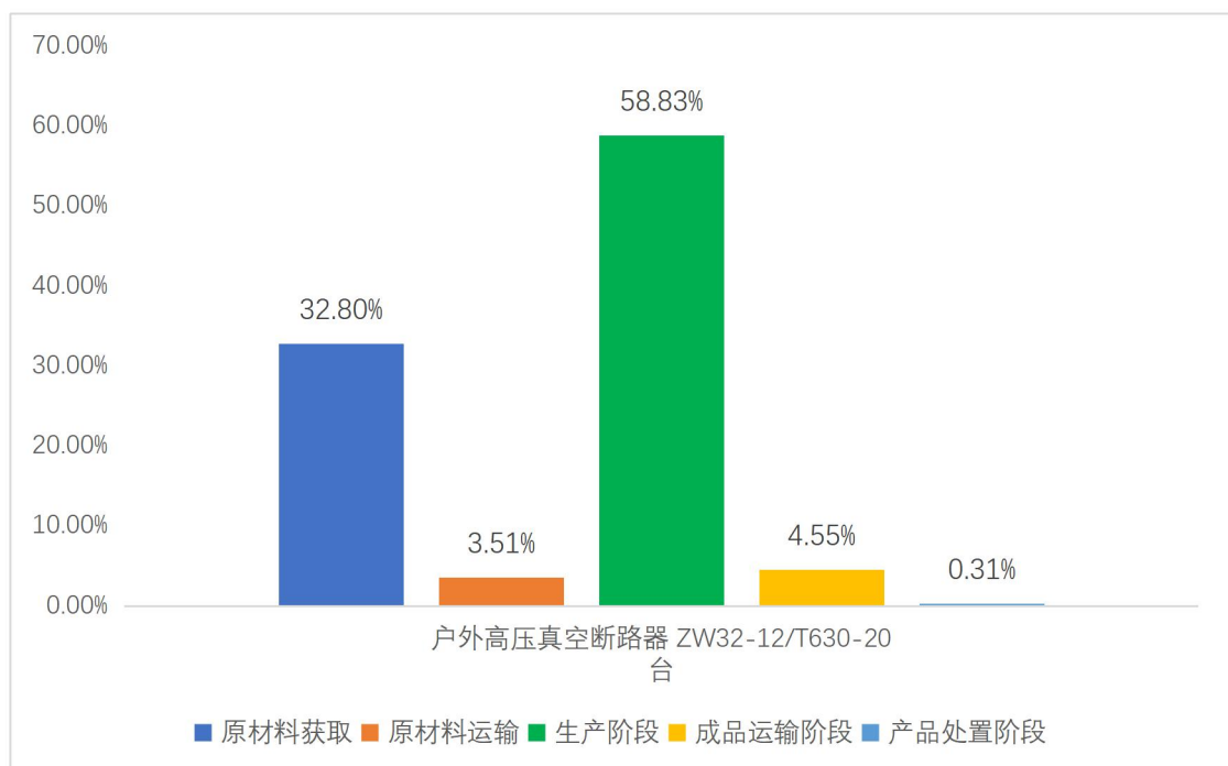
图 5.2.2 户外高压真空断路器：ZW32-12/T630-20 生命周期阶段碳排放分布图
