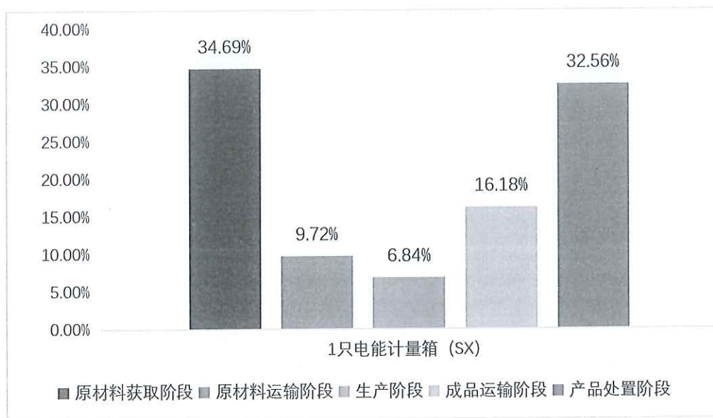
图 5.2-2 一只电能计量箱（SX）生命周期阶段碳排放分布图
