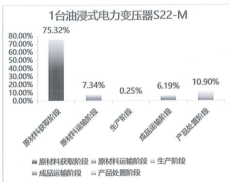
图 5.2-2 一台油浸式电力变压器（S22-M）生命周期阶段碳排放分布图
