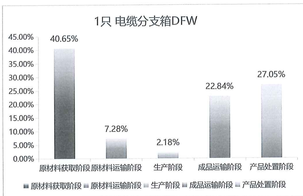
图 5.2-2 一只电缆分支箱（DFW）生命周期阶段碳排放分布图
