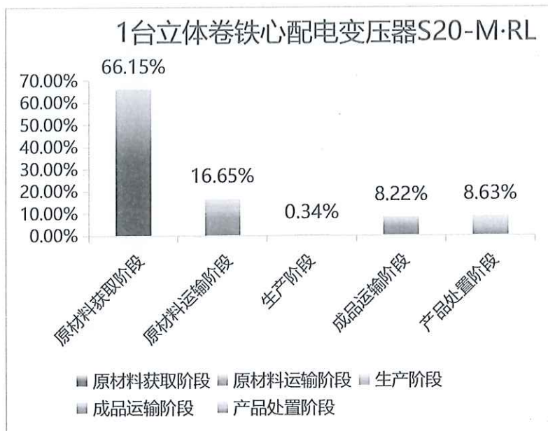
图 5.2-2 一台立体卷铁心配电变压器（S20-M·RL）生命周期阶段碳排放分布图
