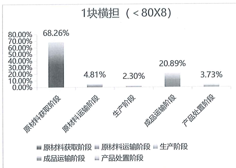
图 5.2-2 1 块横担（<80X8）生命周期阶段碳排放分布图
