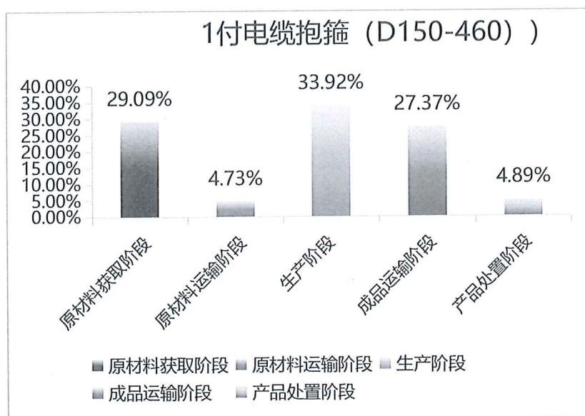
图 5.2-2 1 付电缆抱箍（D150-460）生命周期阶段碳排放分布图
