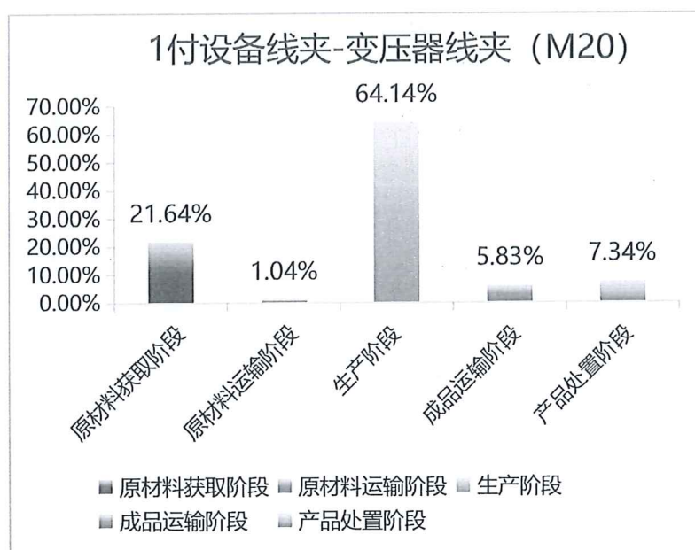
图 5.2-2 1 付设备线夹-变压器线夹（M20）生命周期阶段碳排放分布图
