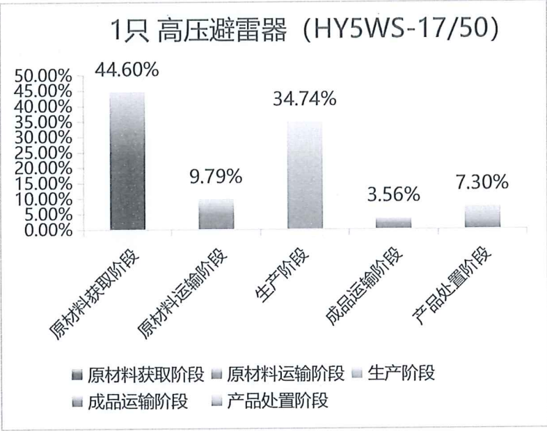
图 5.2-2 1 只高压避雷器（HY5WS-17/50）生命周期阶段碳排放分布图
