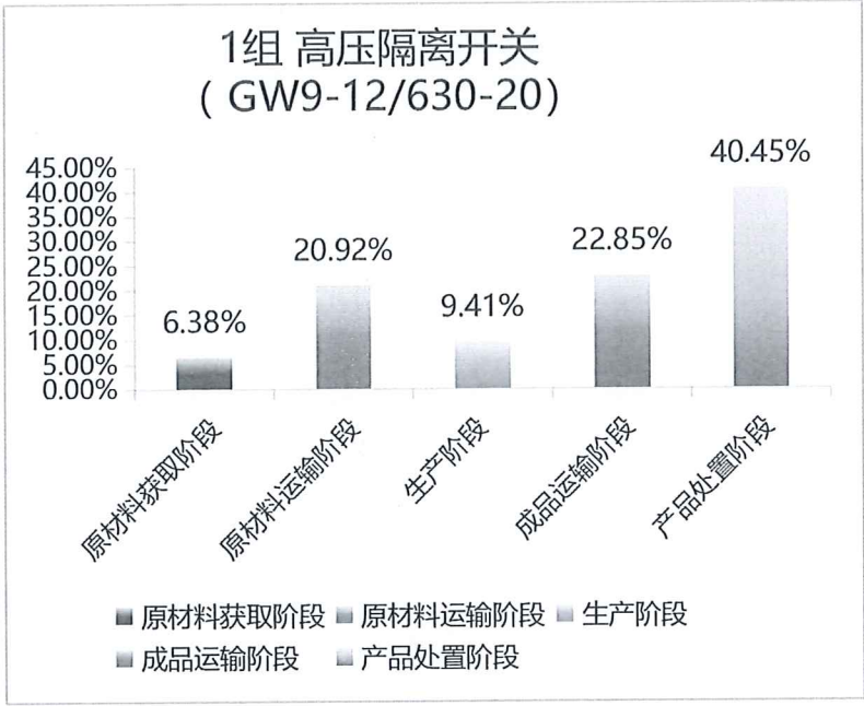
图 5.2-2 1 组高压隔离开关（GW9-12/630-20）生命周期阶段碳排放分布图
