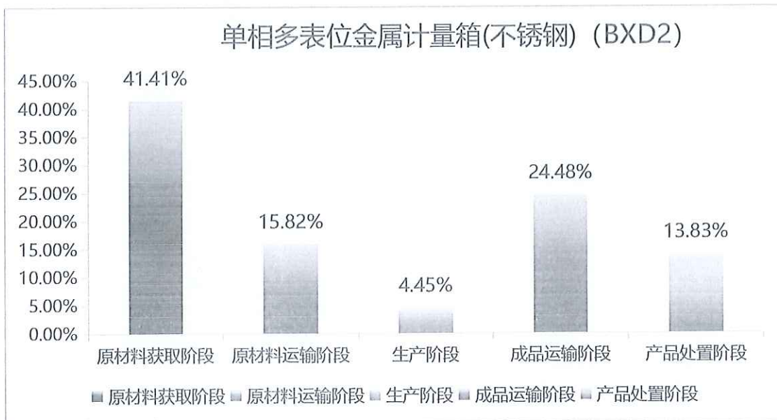
图 5.2-2 一台单相多表位金属计量箱(不锈钢) (BXD2) 生命周期阶段碳排放分布图
