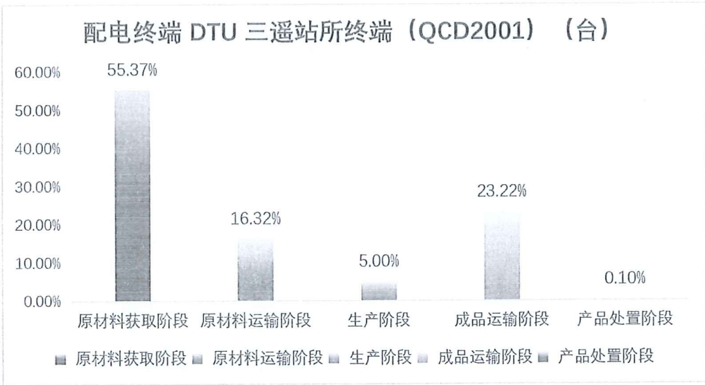
图 5.2-2 1 台配电终端 DTU 三遥站所终端（QCD2001） 产品生命周期阶段碳排放分布图
