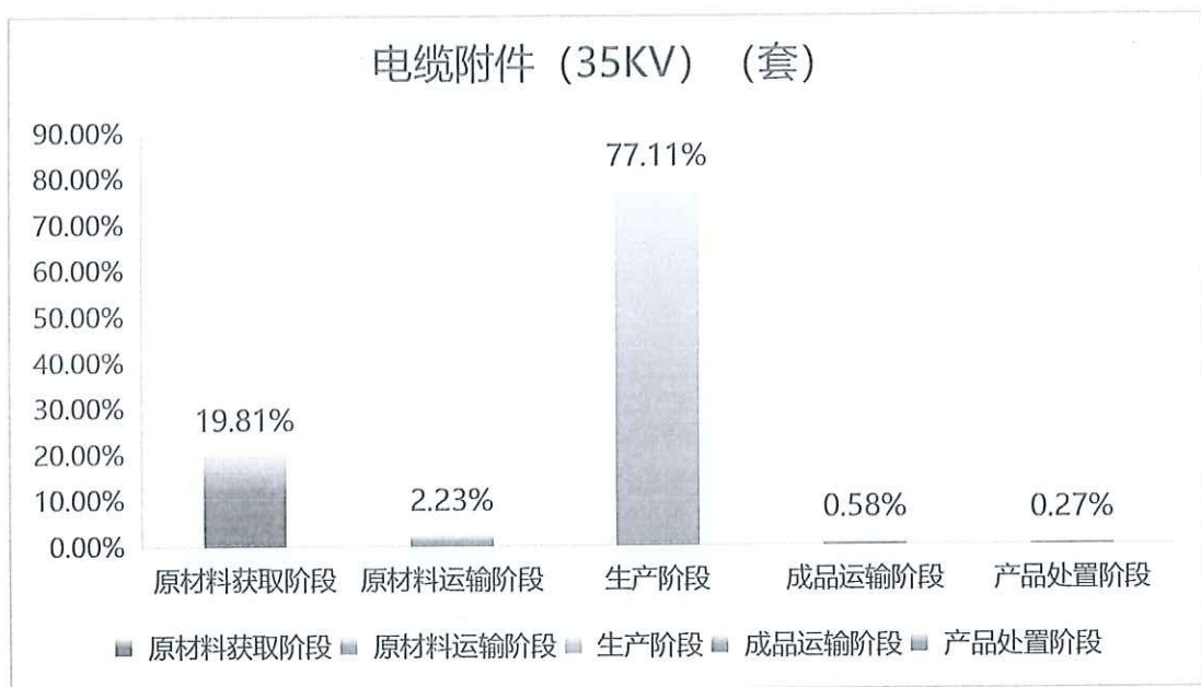
图 5.2-2 一套电缆附件（35KV）生命周期阶段碳排放分布图
