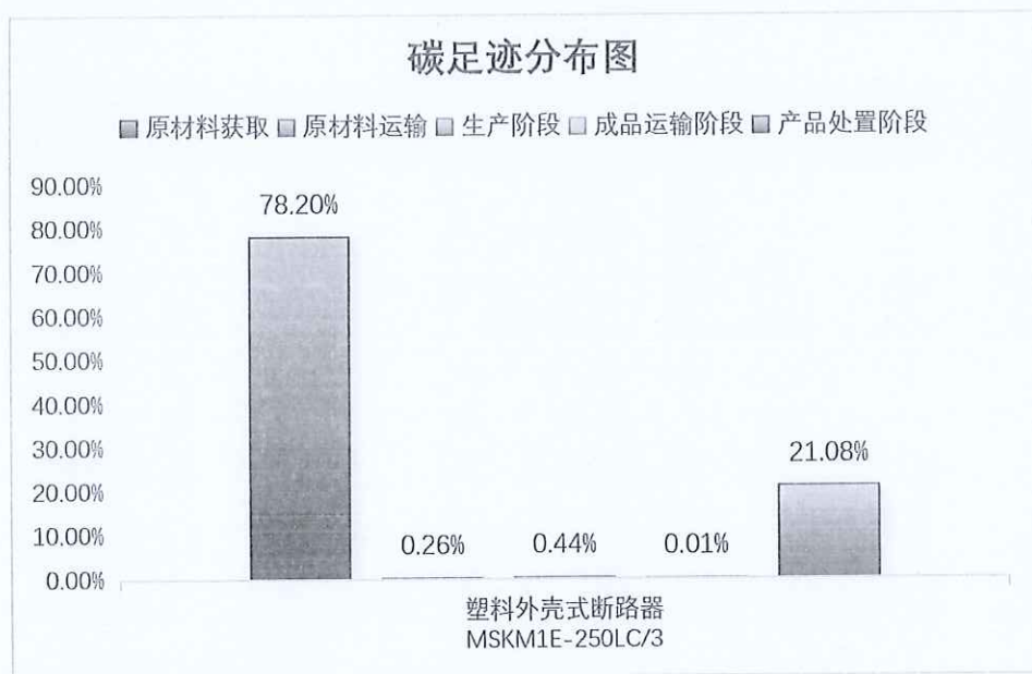
图 5. 2. 1-2 塑料外壳式断路器（MSKM1E-250LC/3）产品生命周期阶段碳排放分布图
