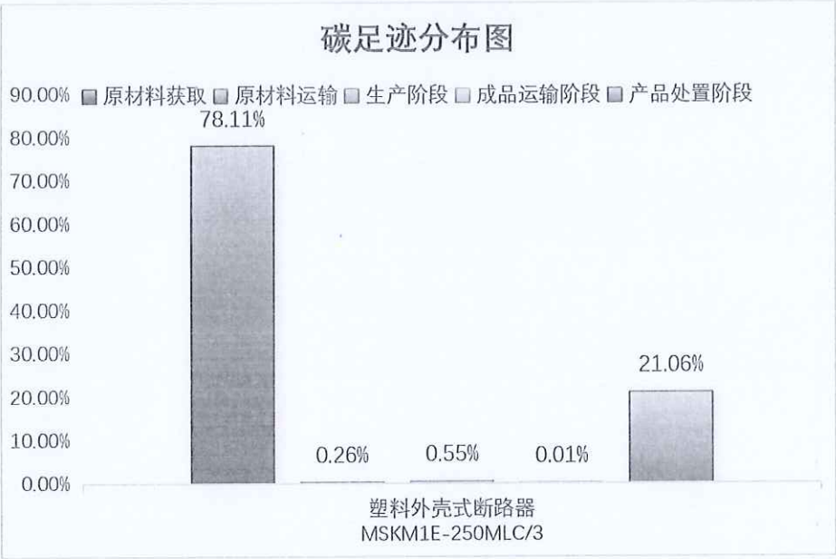
图 5.2.2-2 塑料外壳式断路器（MSKM1E-250MLC/3）产品生命周期阶段碳排放分布图
