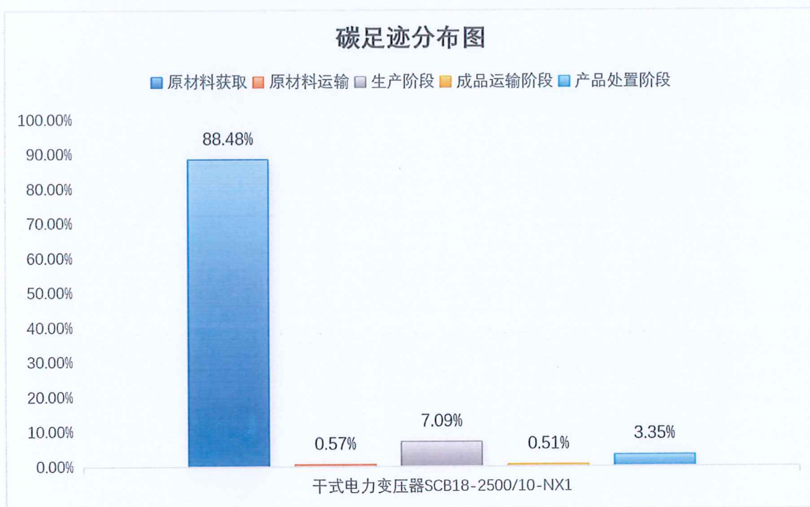
图 5.2.1-2 干式电力变压器（SCB18-2500/10-NX1）产品生命周期阶段碳排放分布图
