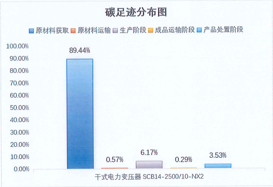
图 5.2.2-2 干式电力变压器（SCB14-2500/10-NX2）产品生命周期阶段碳排放分布图
