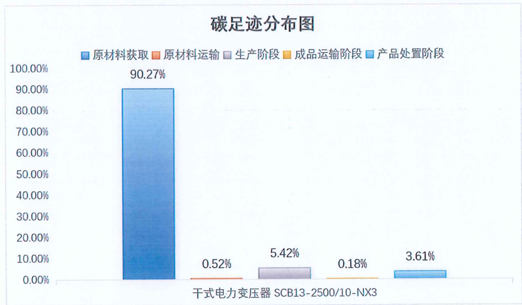
图 5.2.3-2 干式电力变压器（SCB13-2500/10-NX3）产品生命周期阶段碳排放分布图
