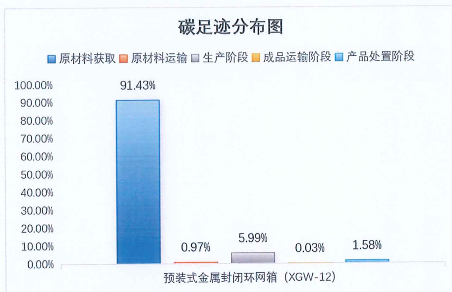
图 5.2-2 预装式金属封闭网箱（XGW-12）产品生命周期阶段碳排放分布图
