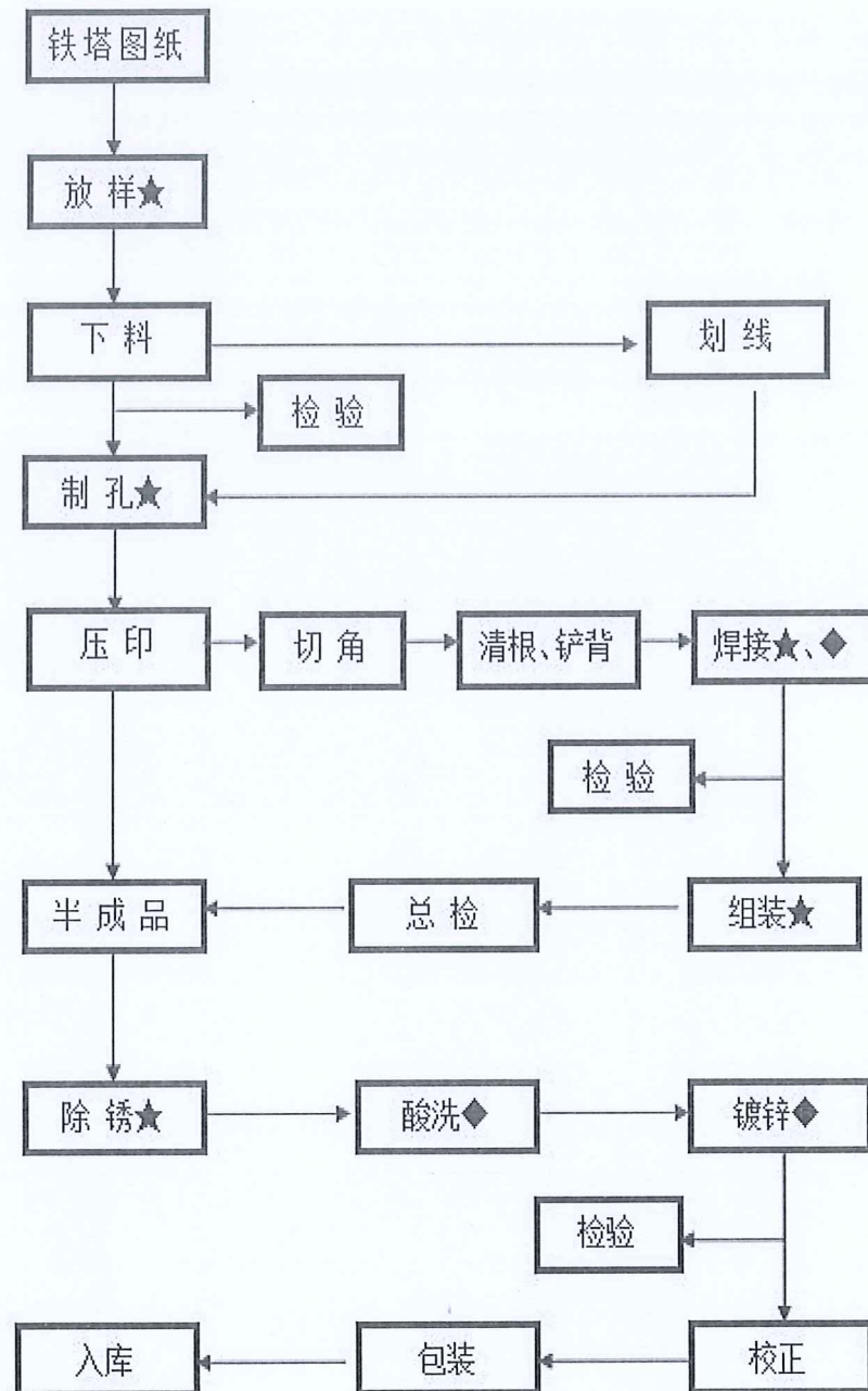
输电线路铁塔生产工艺流程图
