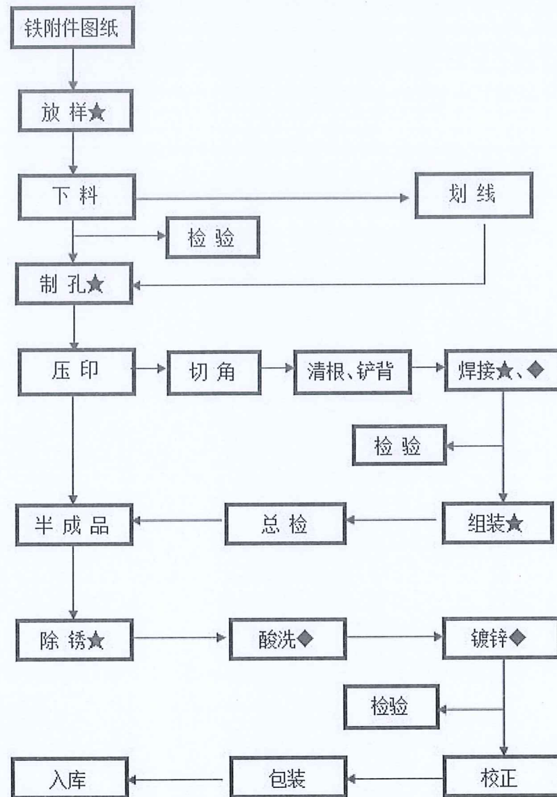
铁附件生产工艺流程图
