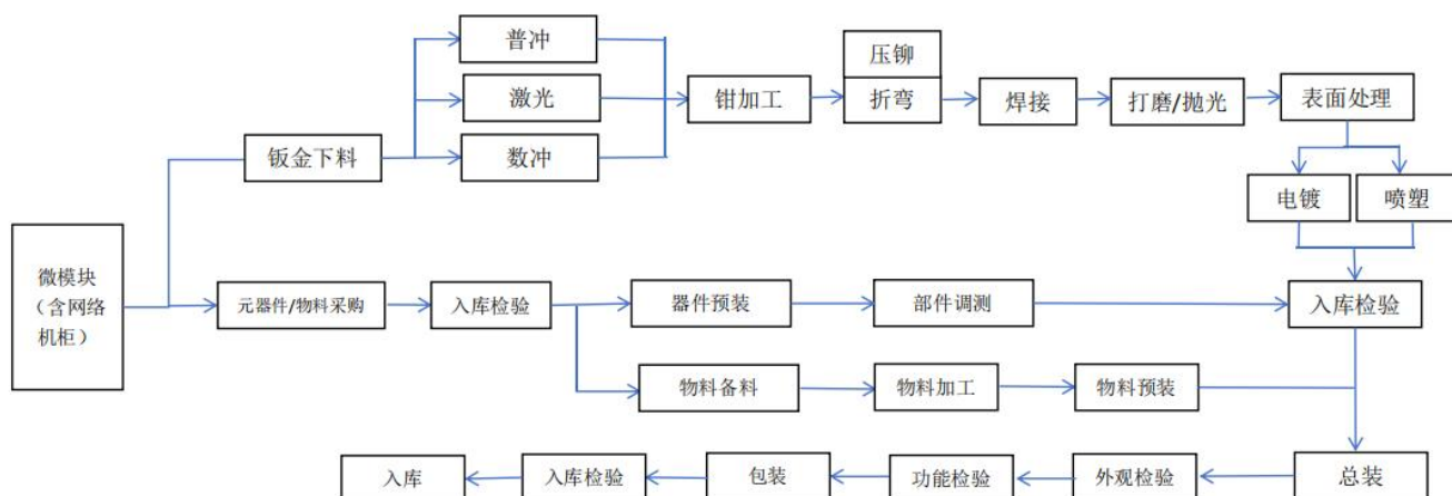
微模块（含网络机柜）制造工艺流程图
