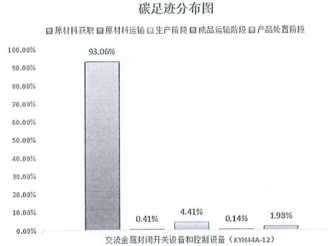
图 5.2-2 交流金属封闭开关设备和控制设备（KYN44A-12）生命周期阶段碳排放分布图
