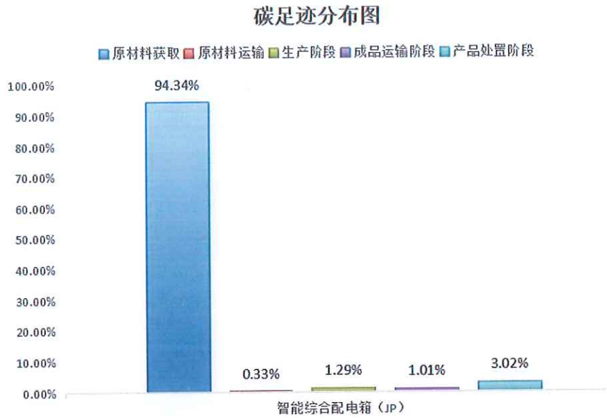
图 5.2-2 智能综合配电箱（JP）生命周期阶段碳排放分布图
