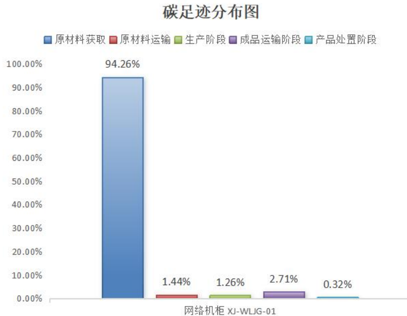
图 5.2-2 网络机柜 XJ-WLJG-01 生命周期阶段碳排放分布图
