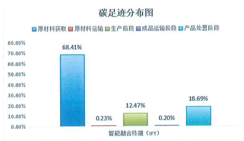
图 5.2-2 智能融合终端（IFT）生命周期阶段碳排放分布图
