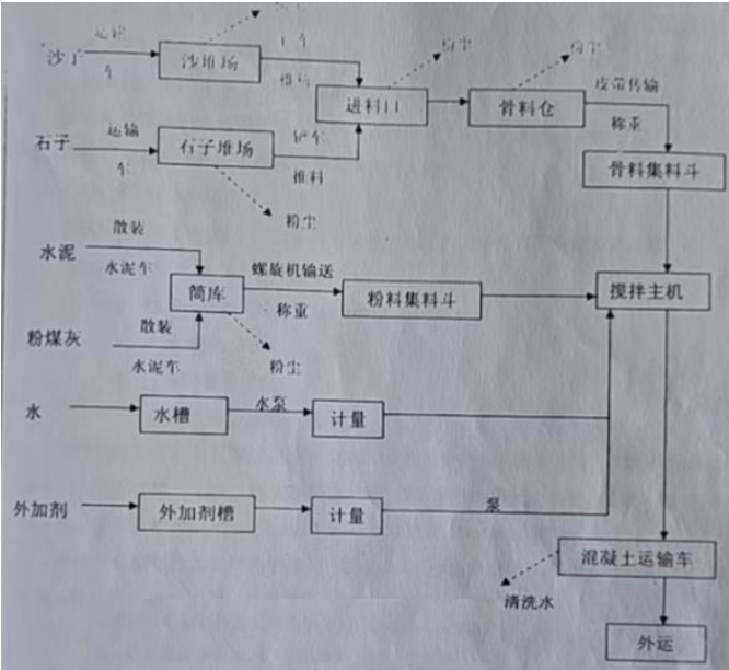
工艺流程图
