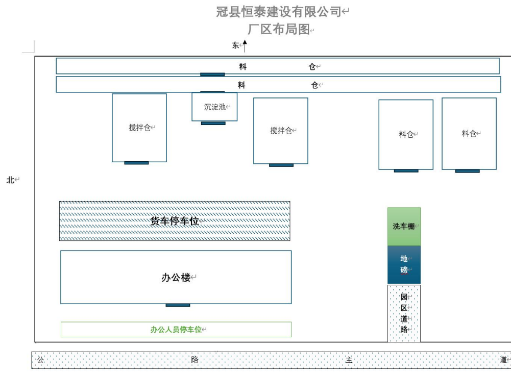
厂区布局图
