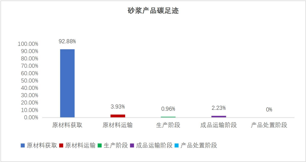
图 5.2-2 砂浆生命周期阶段碳排放分布图
