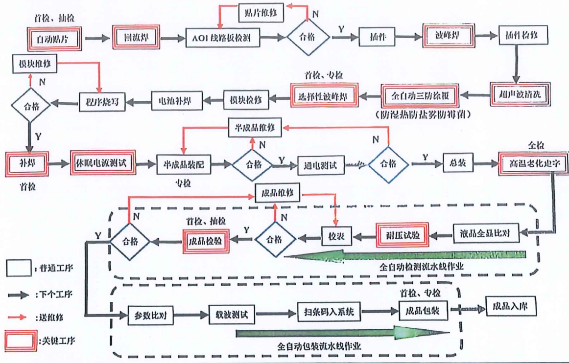
单相费控智能电能表工艺流程图：
