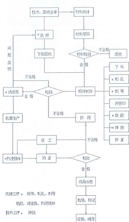
钢管塔工艺流程图
