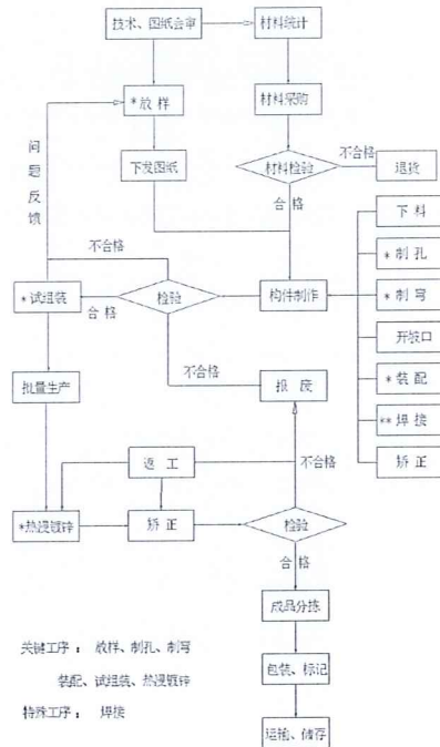
角钢塔工艺流程图
