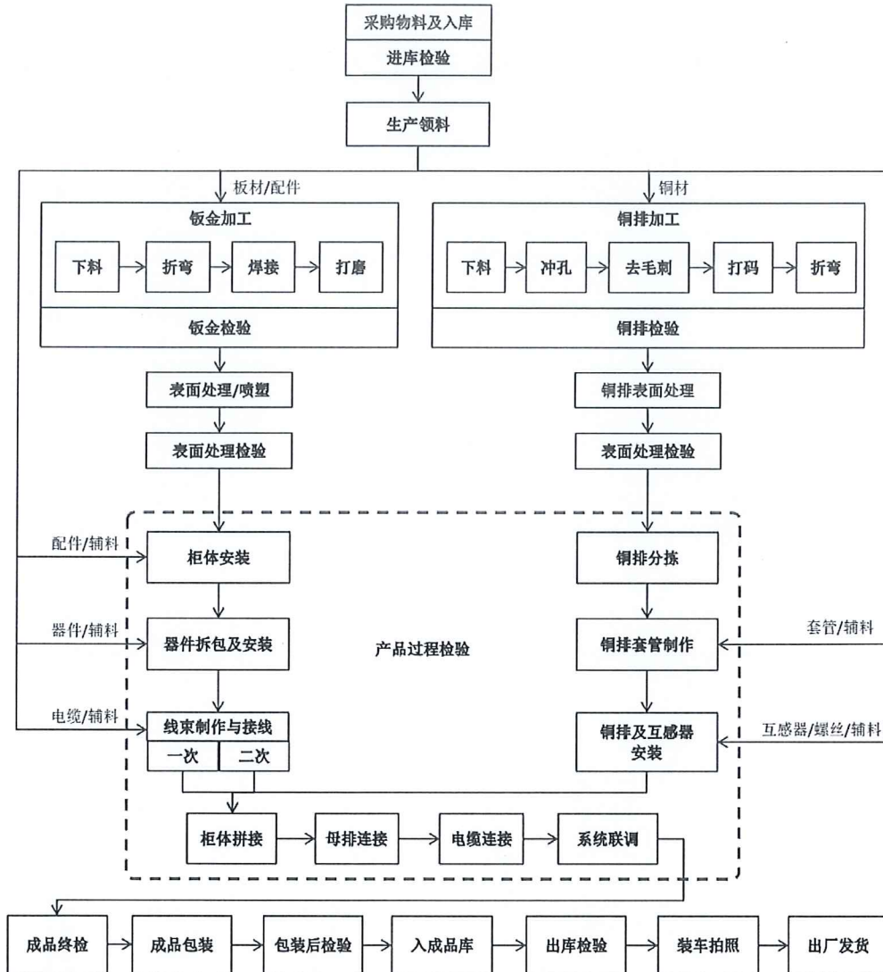
高/低压成套开关设备（包括一体化电力模块）生产工艺流程图
