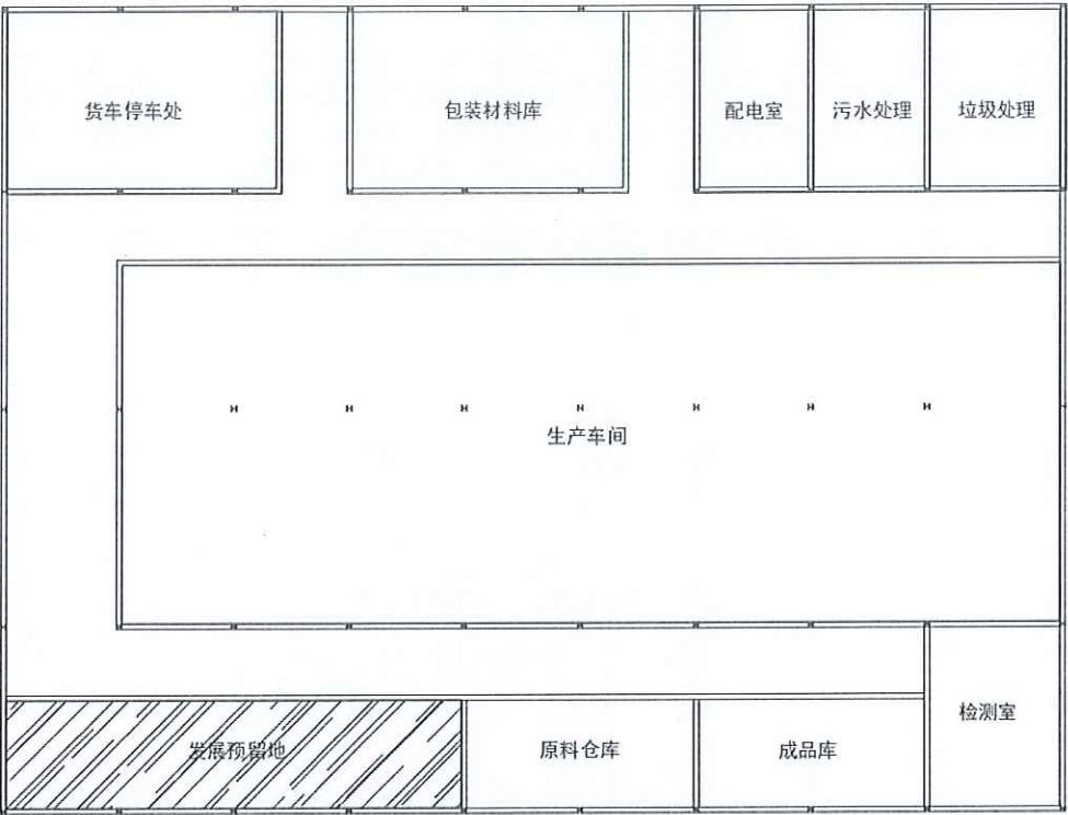
厂区布局图
