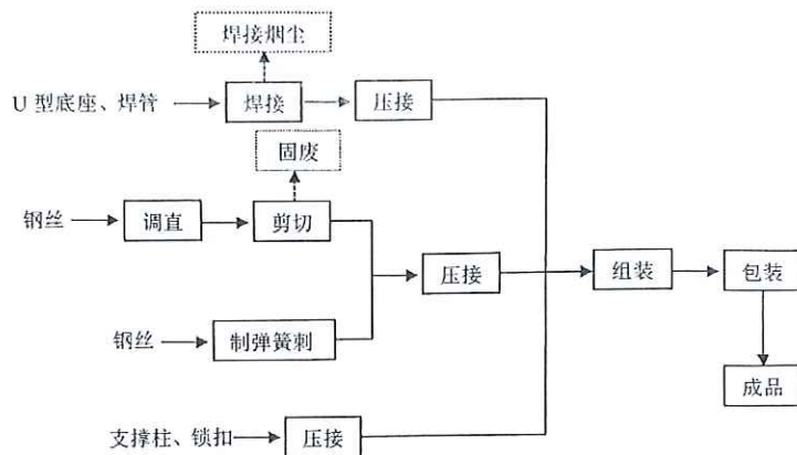
图 2-6 电力金具驱鸟器（防鸟刺）生产工艺流程图
