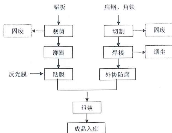
图 2-5 交通、环保标识牌加工工艺流程图
