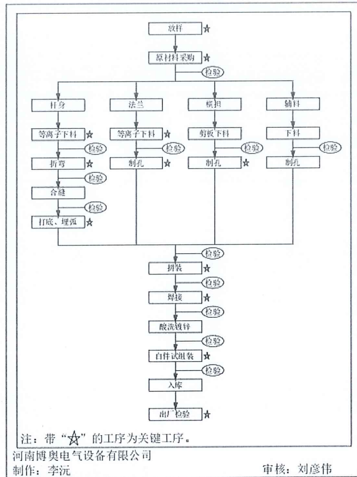
钢管杆生产工艺流程图
